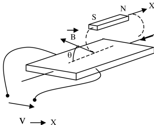
Hình 1-9. Ứng dụng hiệu ứng Hall
