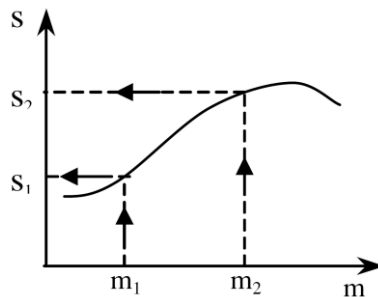
Hình 1-2. Phương pháp chuẩn cảm biến
