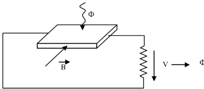
Hình 1-8. Ứng dụng hiệu ứng quang - điện - từ
