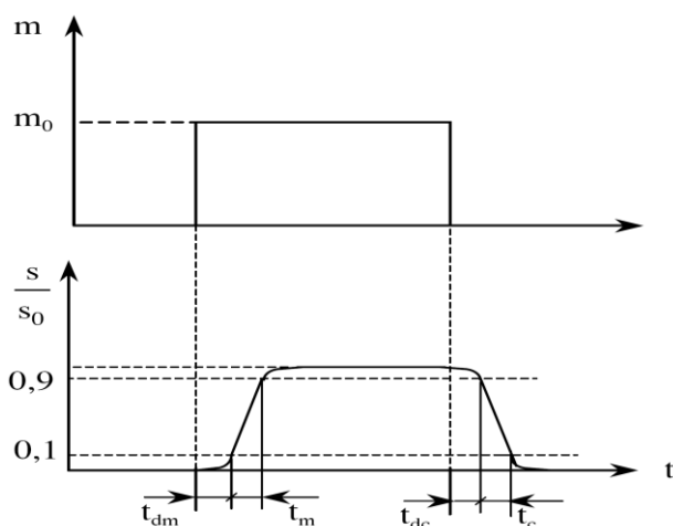
Hình 1-3. Xác định các khoảng thời gian đặc trưng cho chế độ quá độ
