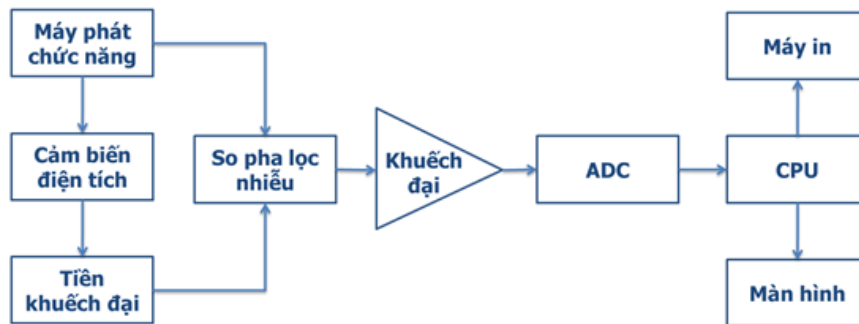
Hình 1-11. Sơ đồ đo điện thế bề mặt
