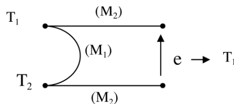
Hình 1-4. Sơ đồ hiệu ứng nhiệt điện
