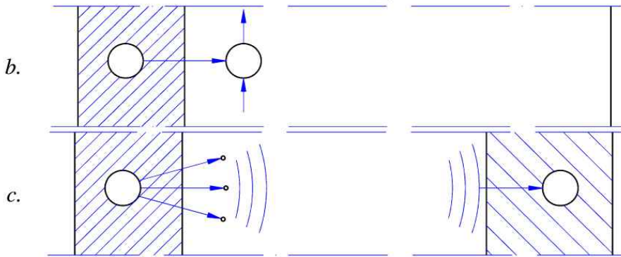
Hình 2.1 Các phương thức trao đổi nhiệt.
