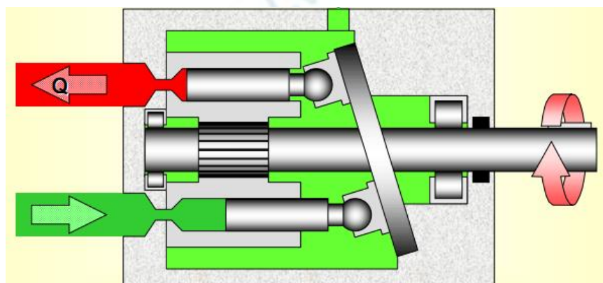
Hình 3.6: Bơm piston hướng trục
