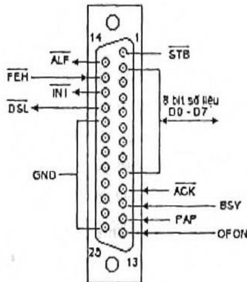
Đầu nối D - 25 cho cổng LPT
