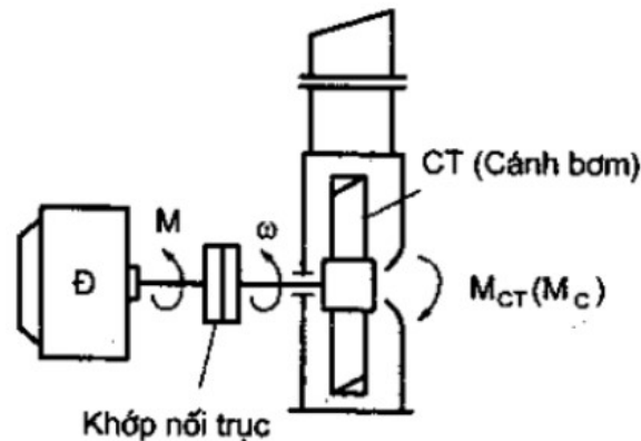
Hình 1. Truyền động của máy bơm nước
