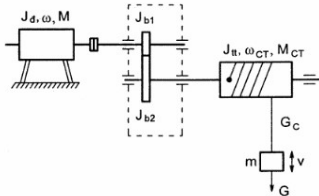
Hình 1-2. Sơ đồ động học của cơ cấu nâng hạ hàng
