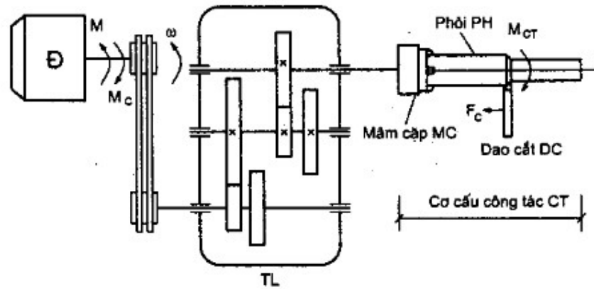
Hình 2. Truyền động mâm cặp máy tiện
