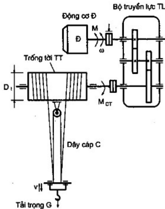
Hình 3. Truyền động của cần trục
