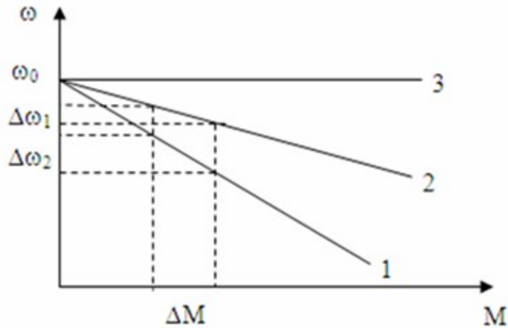
Hình 1-6. Đặc tính cơ của động cơ điện
