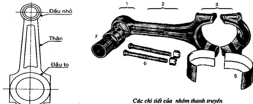
Hình 1.12. Thanh truyền.
