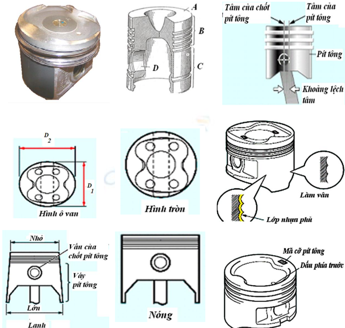
Hình 1.6 Piston.
