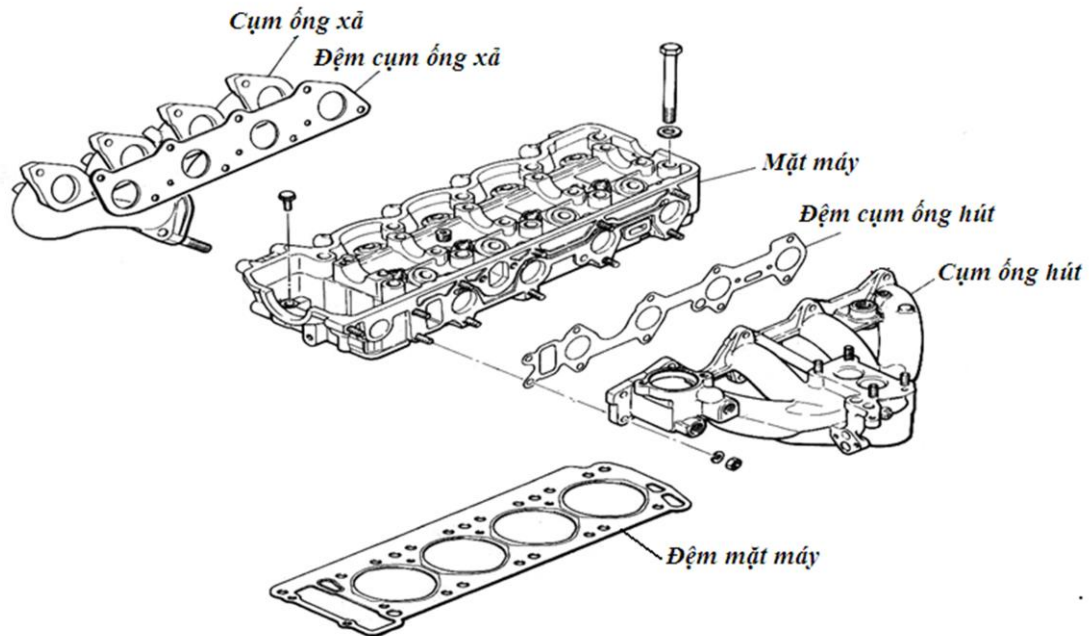
Hình 1.1 Mặt máy.
