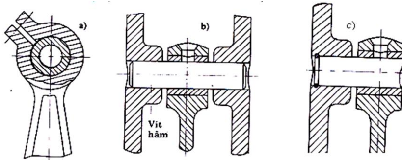
Hình 1.9 Các phương pháp lắp chốt piston.
