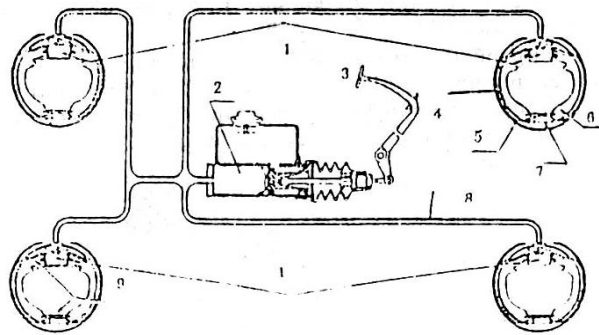
Hình 2.1. Sơ đồ hệ thống phanh thủy lực dẫn động một dòng
