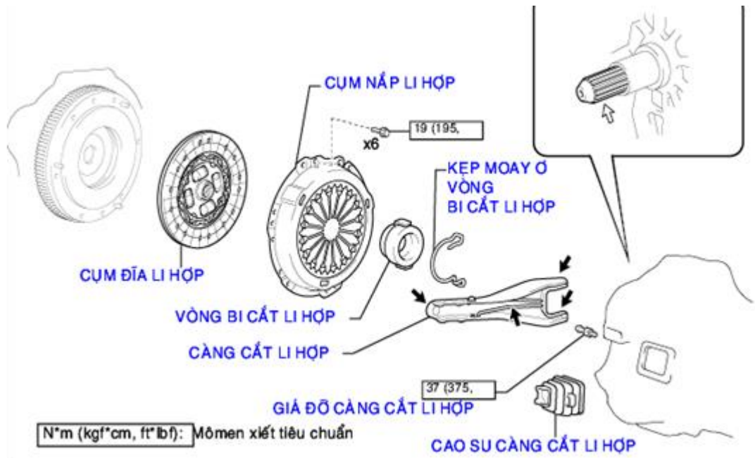
Hình 1.4: Cấu tạo bộ ly hợp
