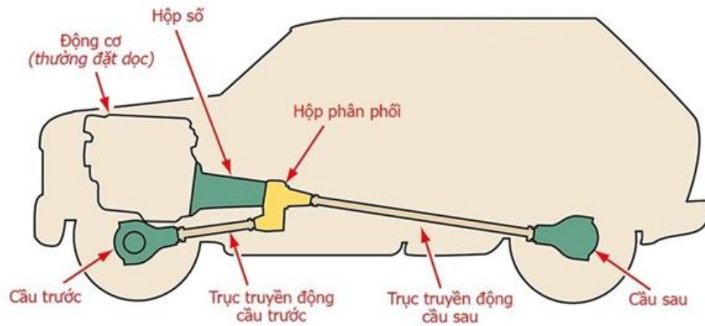
Hình 1.5: Xe có hộp số phụ (hộp phân phối).
