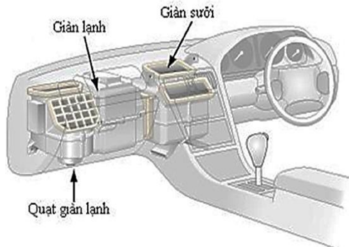
Hình 1.2: Giàn lạnh phía trước
