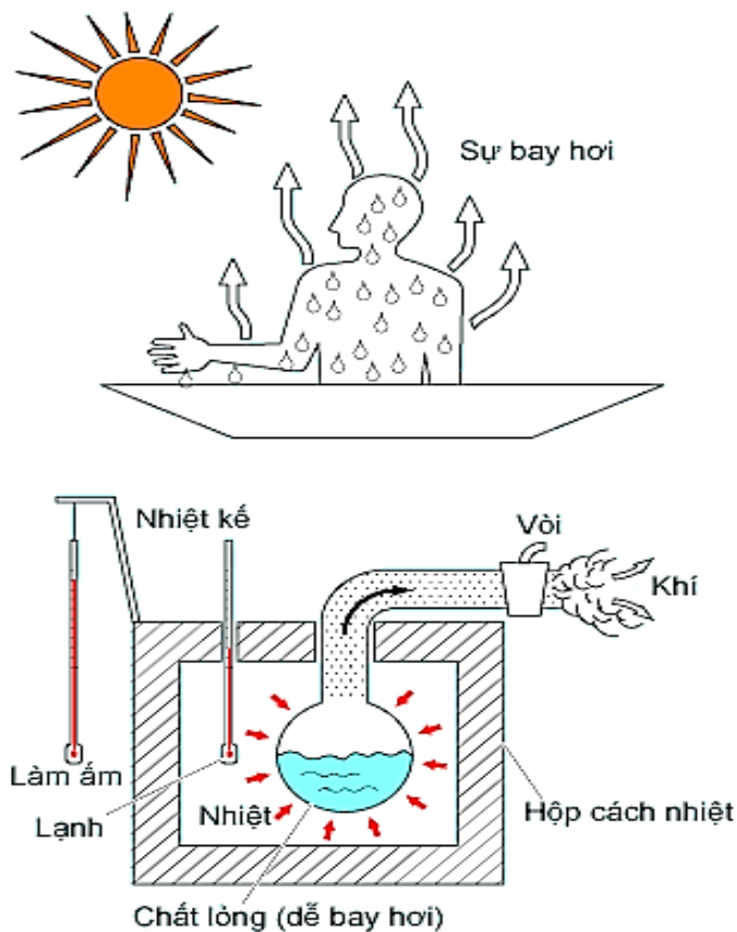
Hình 1.6: Lý thuyết làm lạnh cơ bản
