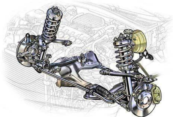
Hình 1.12. Hệ thống treo trước trên ô tô
