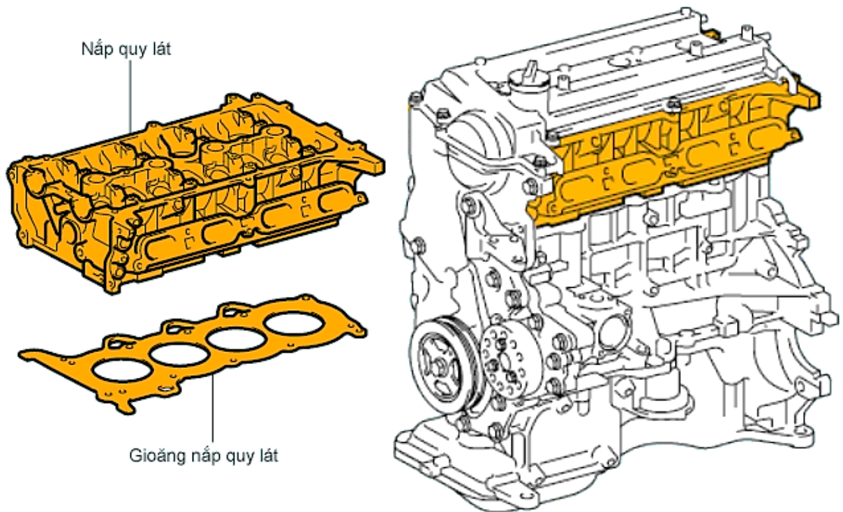
Hình 1.1: Nắp máy động cơ
