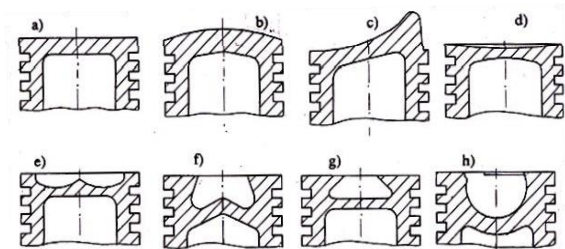
Hình 1.11: Các dạng đỉnh piston
