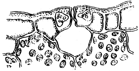
Hình 2.4. Biểu bì
