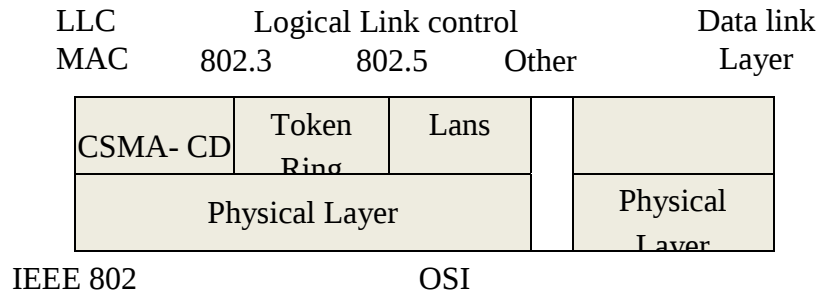
Hình 2.2 - Kiến trúc mạng cục bộ theo IEEE 802
