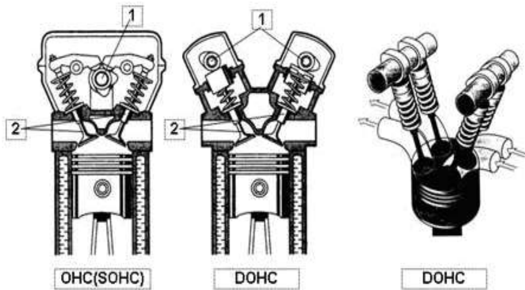
Hình 1.6 Phân biệt SOHC và DOHC
