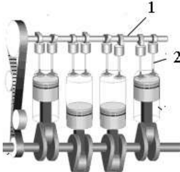
Hình 1.5 Cơ cấu phân phối khí loại trực cam đặt trên nắp máy
