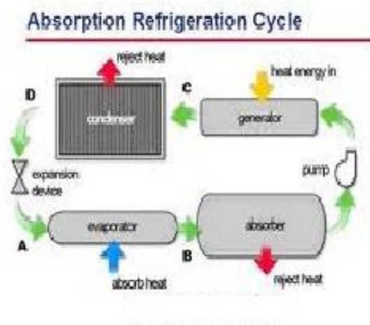
Hình 1.3. Chu trình của máy lạnh hấp thụ
