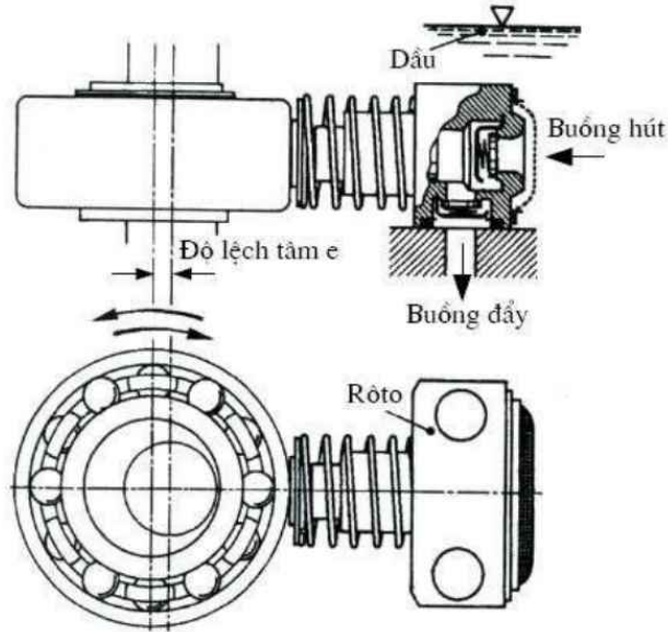
Hình 3.12. Bơm pitton hướng tâm
