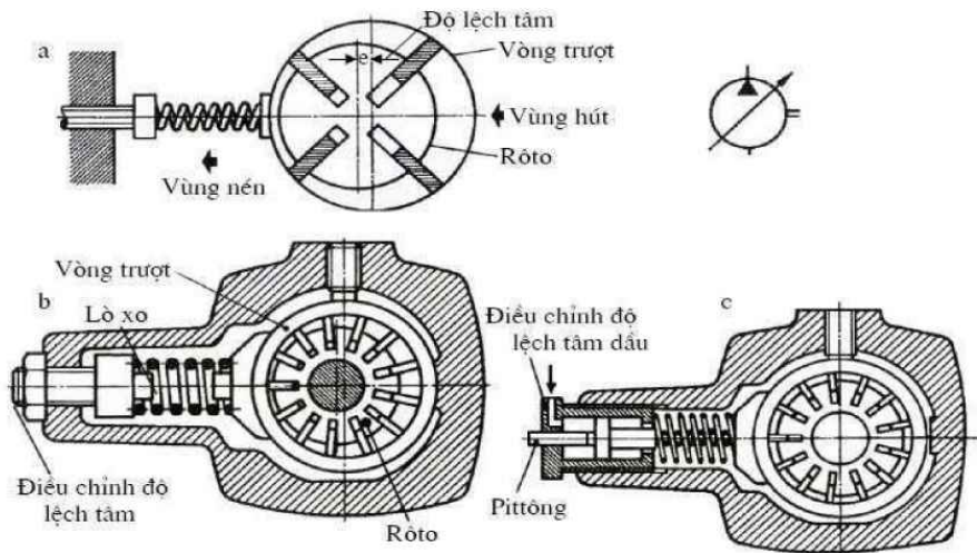
Hình 3.10. Nguyên tắc điều chỉnh lưu lượng bơm cánh gạt đơn a- Nguyên lý và ký hiệu; b- điều chỉnh bằng lò xo; c- Điều chỉnh bằng lưu lượng thủy lực
