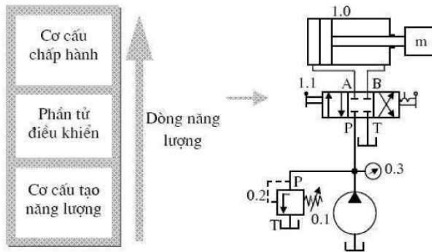
Hình 3.2. Sơ đồ cấu trúc hệ thống điều khiển bằng thủy lực 1.2. Yêu cầu
