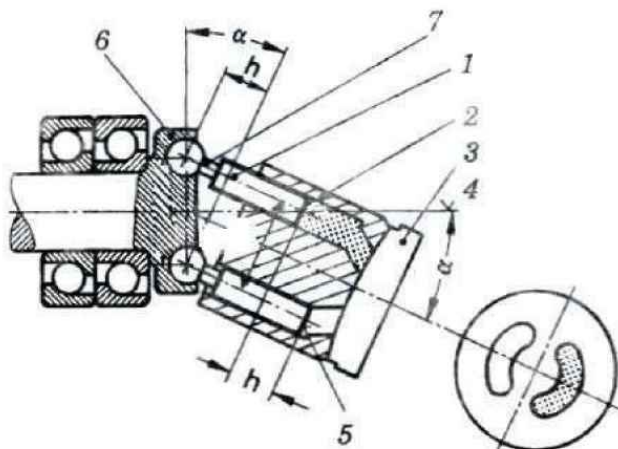
Hình 3.13. Bơm pitton hoặg trực
