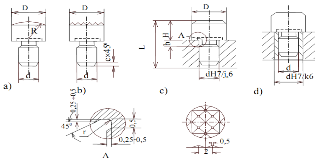
Hình 2- 1: Các loại chốt tì cố định
