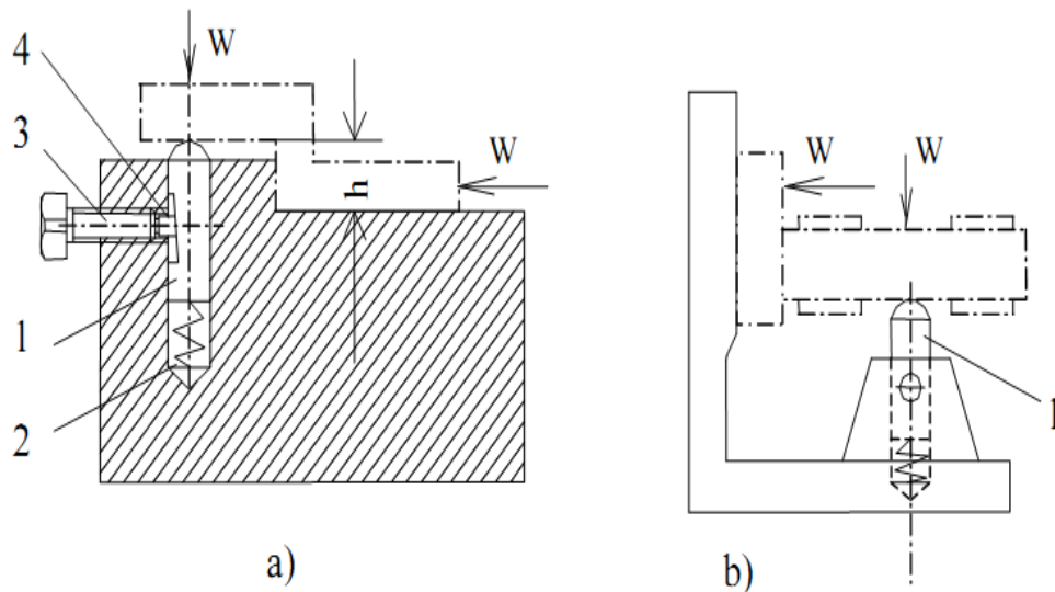
Hình 2-4 : Chốt tì phụ
