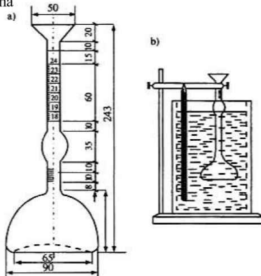
Hình 1-1: Bình tỉ trọng
