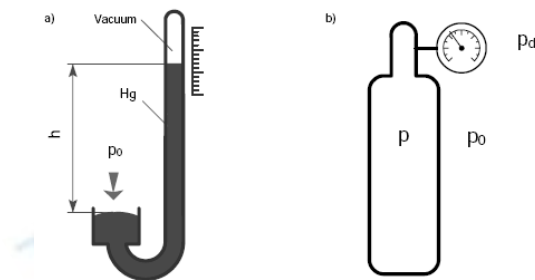
Hình 1.5: Dụng cụ đo áp suất
