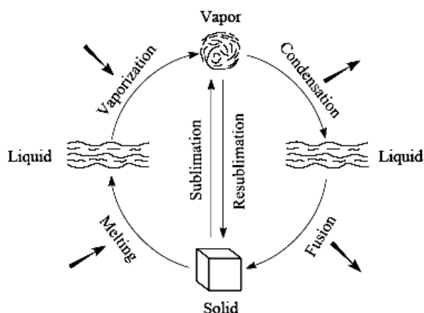
Hình 1.8: Các quá trình chuyển pha của nước
