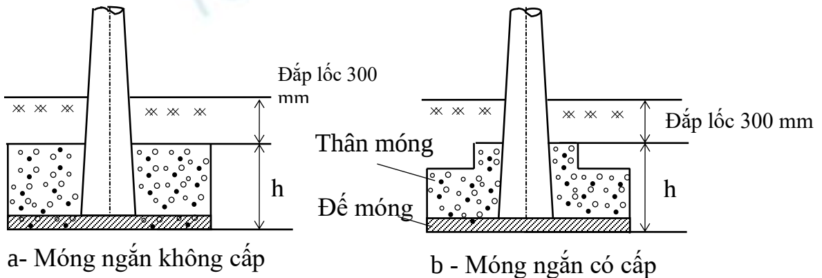
Hình 1-4. Móng ngắn
