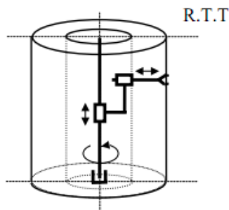
Hình 1.2 – Robot kiểu tọa độ trụ
