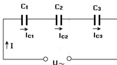
Hình 1.13: Tụ điện mắc nối tiếp trong mạch.
