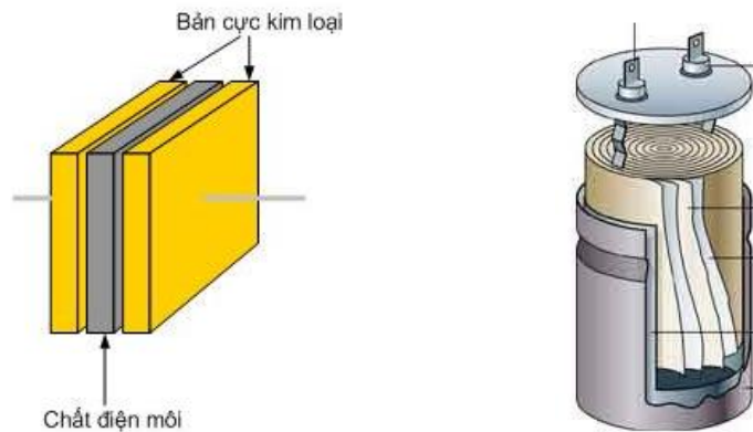
Hình 1.16 : Cấu tạo tụ gốm và tụ hoá
