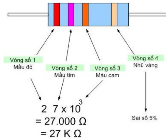
Hình 1.8: Điện trở 4 vòng màu và cách đọc.
