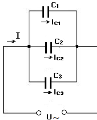
Hình 1.14: Tụ điện mắc song song.
