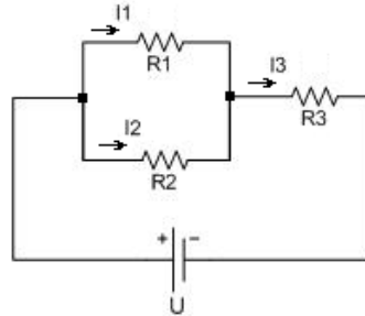
Hình 1.3: Điện trở mắc hỗn hợp trong mạch.
