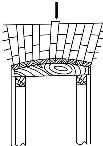
Hình 5.1: Xây gạch nghiêng qua khoảng trống
