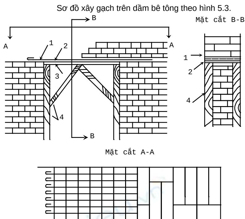
Hình 5.2 Xây gạch nằm qua khoảng trống
