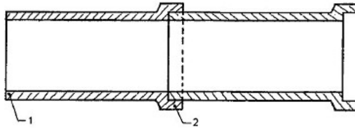
Hình 1 - Khớp nối
