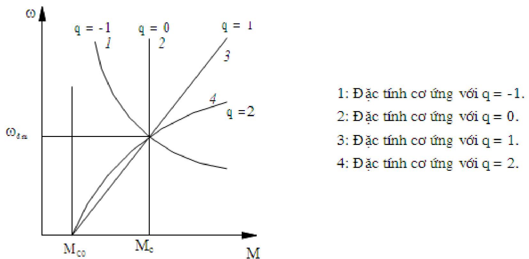
Hình 1-7. Đặc tính cơ của cơ cấu sản xuất ứng với các trường hợp máy sản xuất khác nhau.
