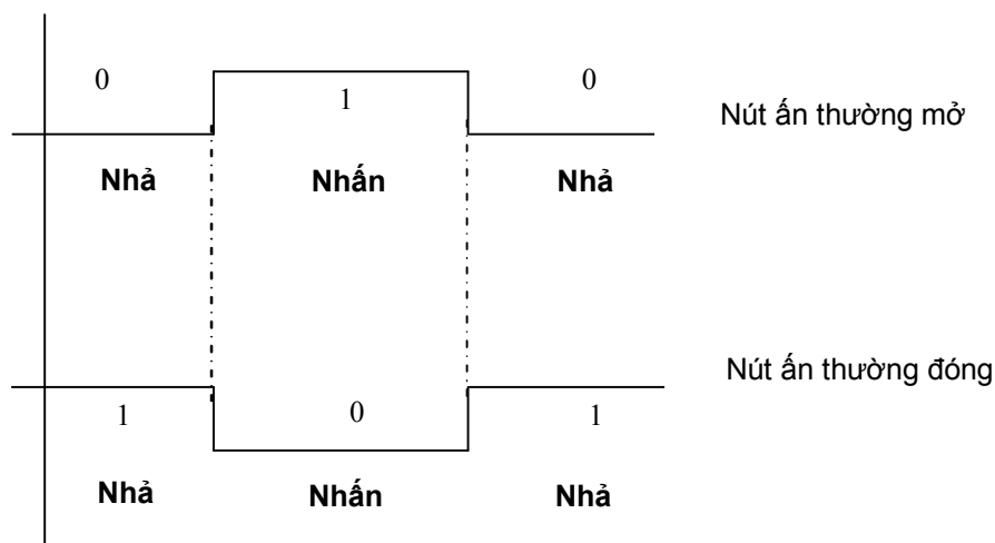
HÌNH 1.5: TÍN HIỆU DO NÚT ẤN TẠO RA
