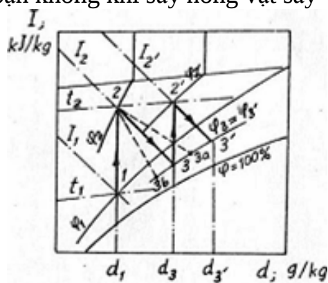
Hành 3.9 Quá trình sấy.
