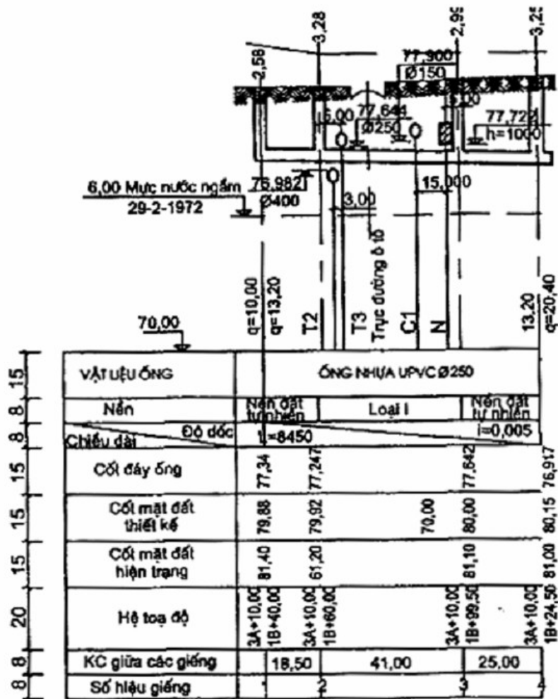
Hình 3 - Ví dụ thể hiện mặt cắt mạng lưới cấp thoát nước trong nhà
