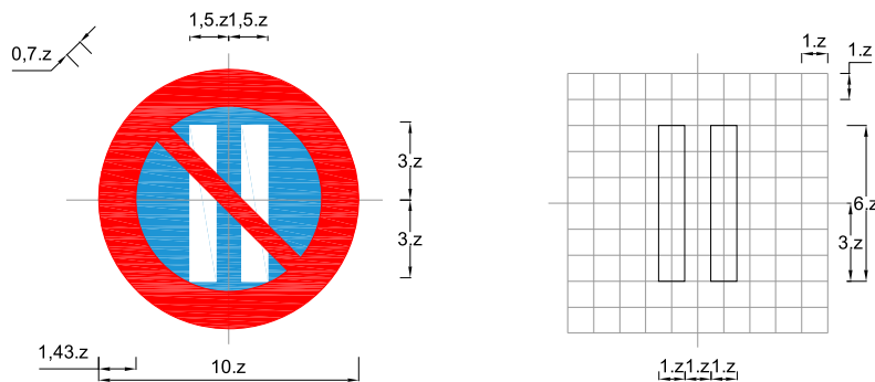
Biển số P.131c: Cấm đỗ xe vào ngày chẵn
