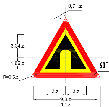
Biển số W.218: Cửa chui
