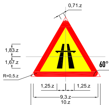
Biển số W.238: Đường cao tốc phía trước
