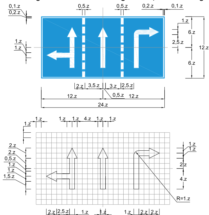
Biển số R.412a: Làn đường dành cho xe ô tô khách
