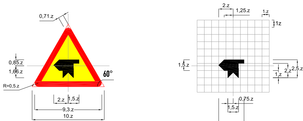
Biển số W.207h: Giao nhau với đường không ưu tiên
