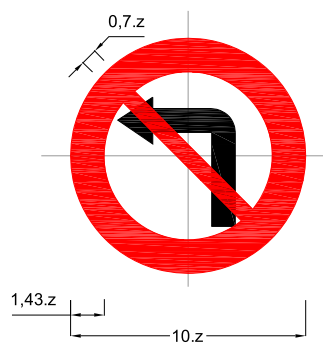
Biển số P.123a: Cấm rẽ trái
