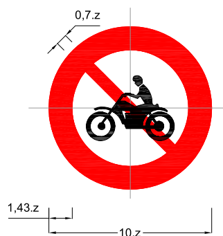
Biển số P.104: Cấm xe mô tô
