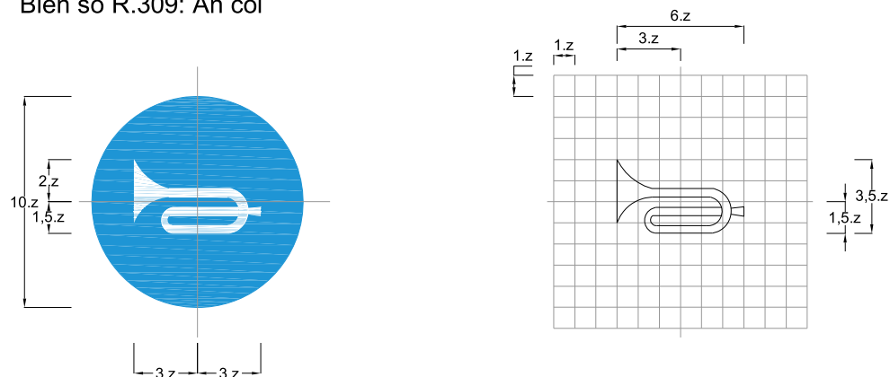
Biển số R.309: Ấn còi
