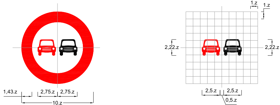
Biển số P.125: Cấm vượt
