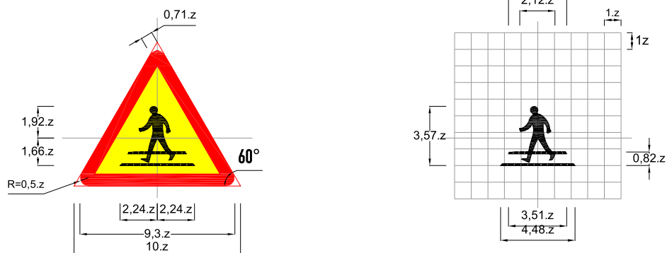
Biển số W.224: Đường người đi bộ cắt ngang
