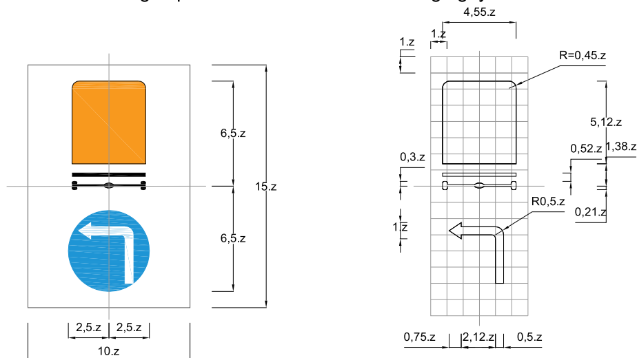
Biển số R.310b: Hướng đi phải theo cho các xe chở hàng nguy hiểm
