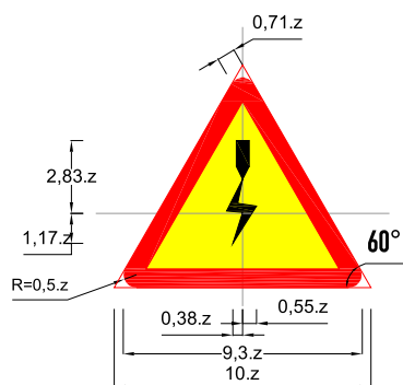
Biển số W.239: Đường cáp điện ở phía trên
