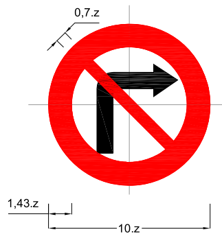
Biển số P.123b: Cấm rẽ phải
