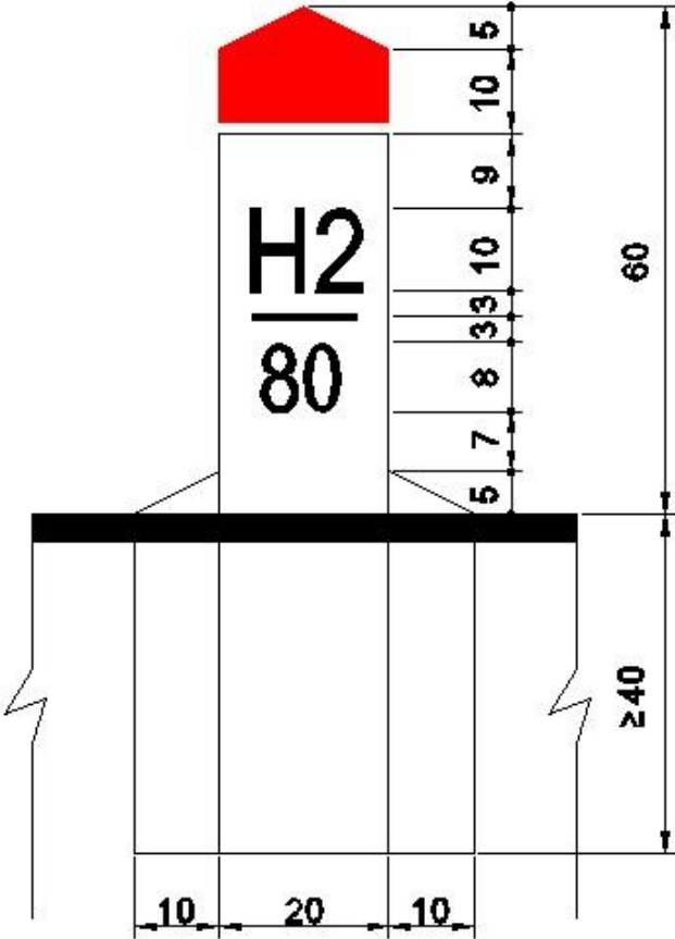
Ghi chú: Kích thước ghi trên hình vẽ là cm Hình I.6 – Chi tiết cọc H
