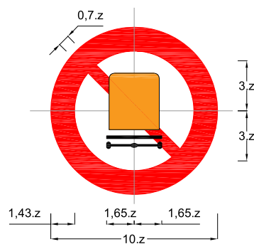
Biển số P.106c: Cấm xe chở hàng nguy hiểm
