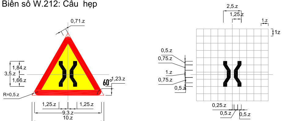
Biển số W.212: Cầu hẹp
