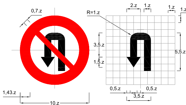
Biển số P.124a: Cấm quay đầu xe
