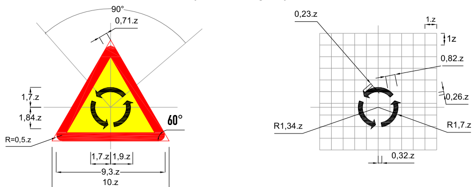
Biển số W.206: Giao nhau chạy theo vòng xuyên
