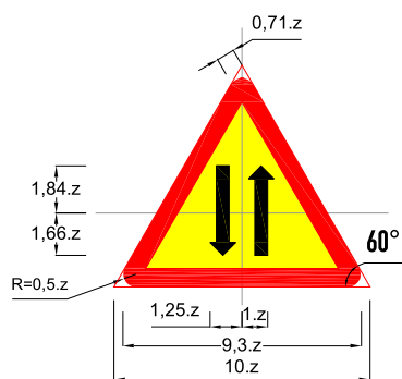
Biển số W.204: Đường hai chiều
