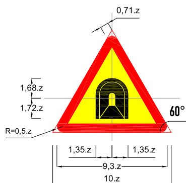
Biển số W.240: Đường hầm
