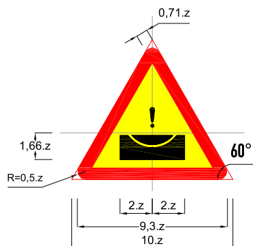
Biển số W.216b: Đường ngầm có nguy cơ lũ quét
