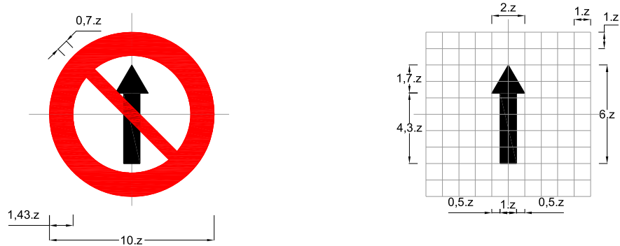
Biển số P.136: Cấm đi thẳng
