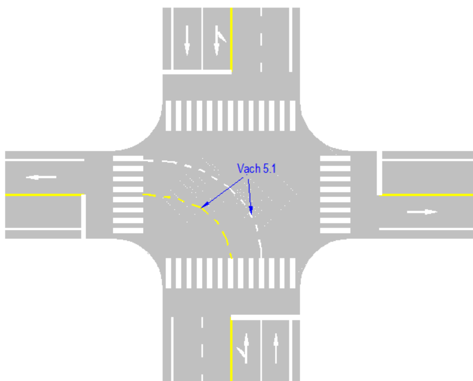
Hình G.40 - Minh họa bố trí vạch 5.1
