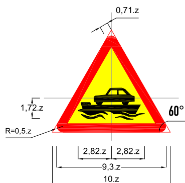
Biển số W.217: Bến phà
