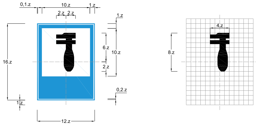
Biển số I.427b : Trạm kiểm tra tải trọng xe
