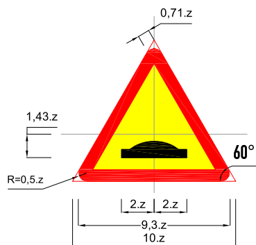
Biển số W.221b: Đường có gồ giảm tốc
