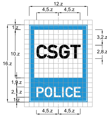
Biển số I.436 : Trạm cảnh sát giao thông
