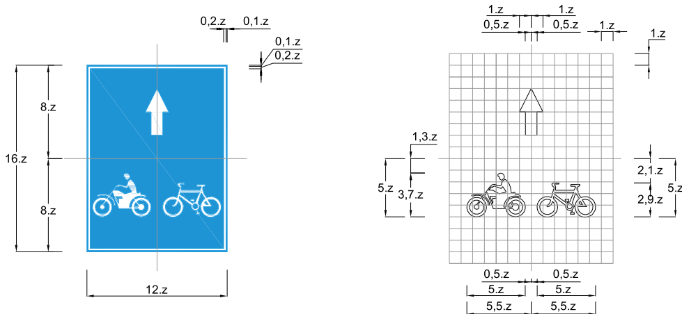
Biển số R.412g: Làn đường dành cho xe máy và xe đạp
