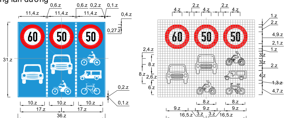
Biển số P.127c: Biển gộp tốc độ tối đa cho phép theo phương tiện trên từng làn đường
