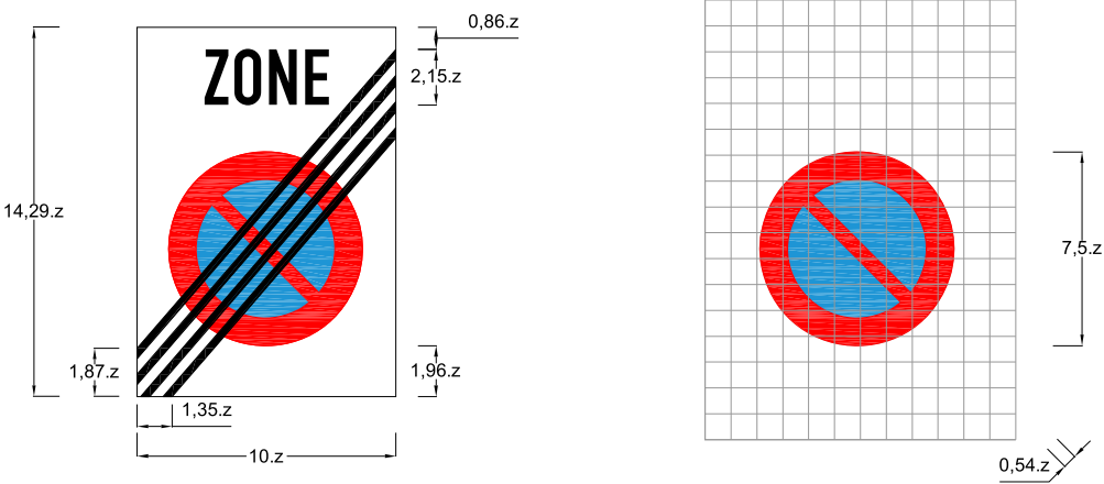
Biển số R.E,10b: Hết cấm đỗ xe theo giờ trong khu vực
