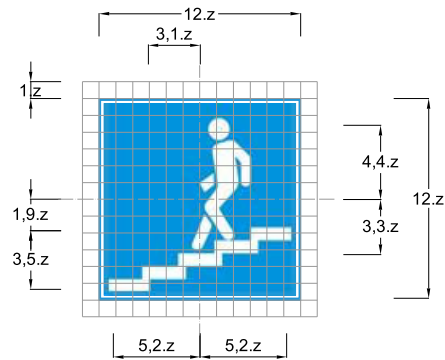
Biển số I.424d : Hàm chui qua đường cho người đi bộ
