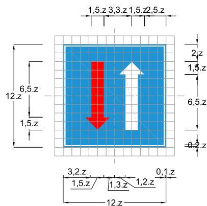
Biển số I.406: Được ưu tiên qua đường hẹp (Priority at narrow road)
