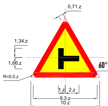
Biển số W.205b: Đường giao nhau
