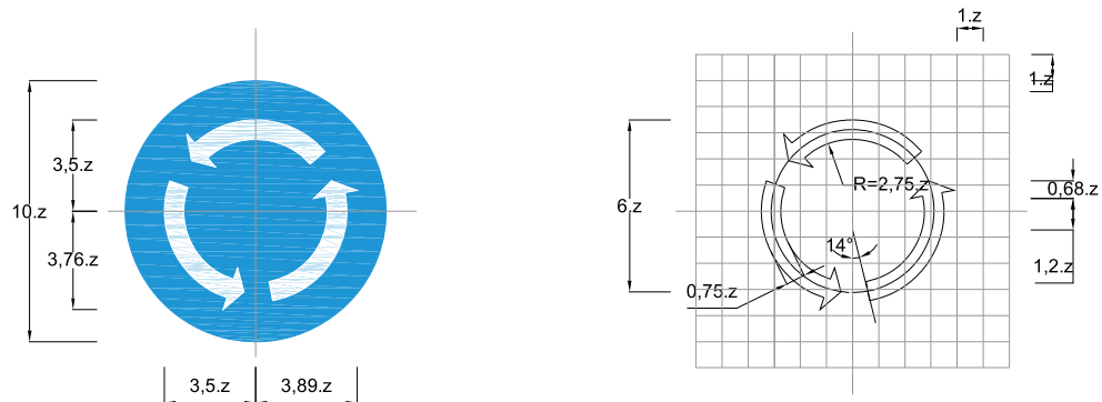
Biển số R.303: Nơi giao nhau chạy theo vòng xuyến
