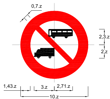
Biển số P.107: Cấm xe ô tô khách và xe ô tô tải
