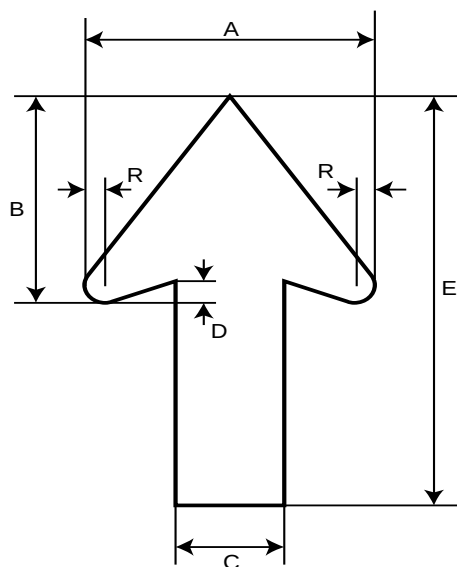
Kích thước mũi tên
