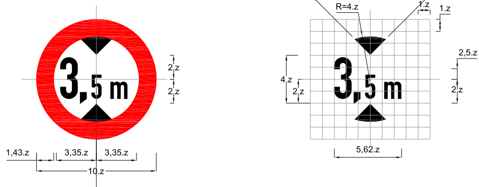
Biển số P.117: Hạn chế chiều cao
