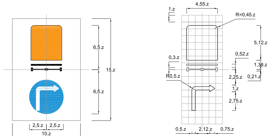
Biển số R.310c: Hướng đi phải theo cho các xe chở hàng nguy hiểm
