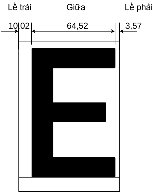
Hình K.1 – Ký hiệu các chi tiết kích thước chữ
