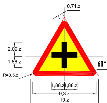
Biển số W.205a: Đường giao nhau
