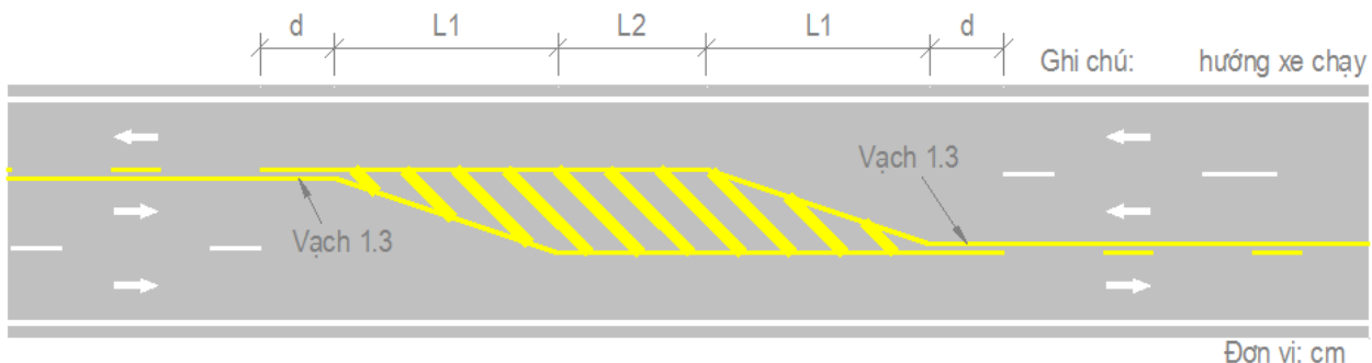
Hình G.8 - Bố trí vạch sơn phân chia hai chiều xe chạy cho đường có 3 làn xe trong khu vực số làn trên một hướng thay đổi từ một làn sang hai làn
