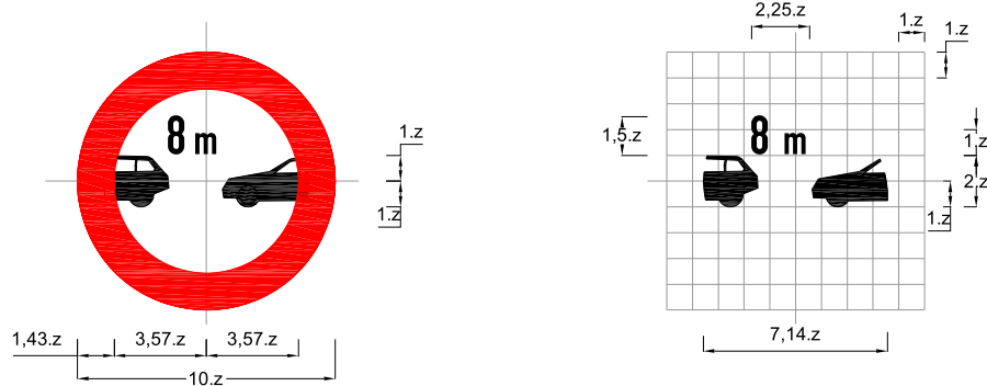
Biển số P.121: Cự ly tối thiểu giữa hai xe
