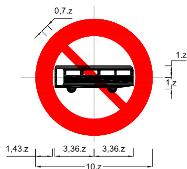
Biển số P.107a: Cấm xe ô tô khách
