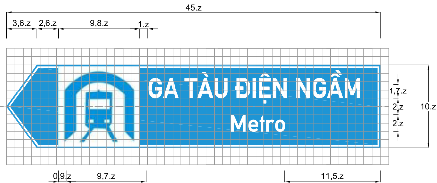
Biển số I.444k : Biển báo chỉ dẫn địa điểm
