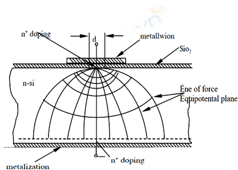
Hình 1.7 Cấu trúc cơ bản của cảm biến Silic
