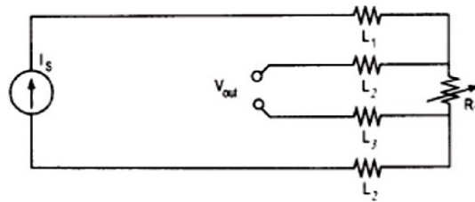
Hình 1.6 Kỹ thuật nối 4 dây
