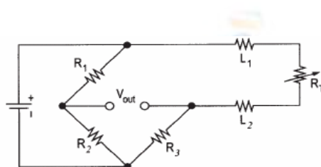
Hình 1.4 Kỹ thuật nối 2 dây
