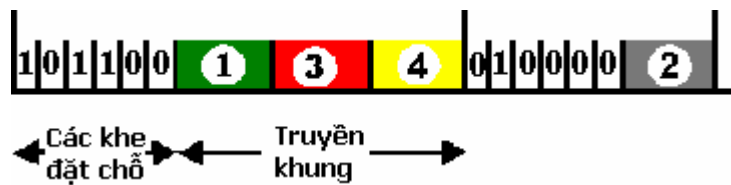
H5.14 Mô tả các chu kỳ hoạt động của hệ thống Thăm dò phân tán
