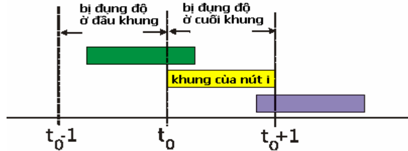
H5.8 Minh họa giao thức Pure ALOHA
