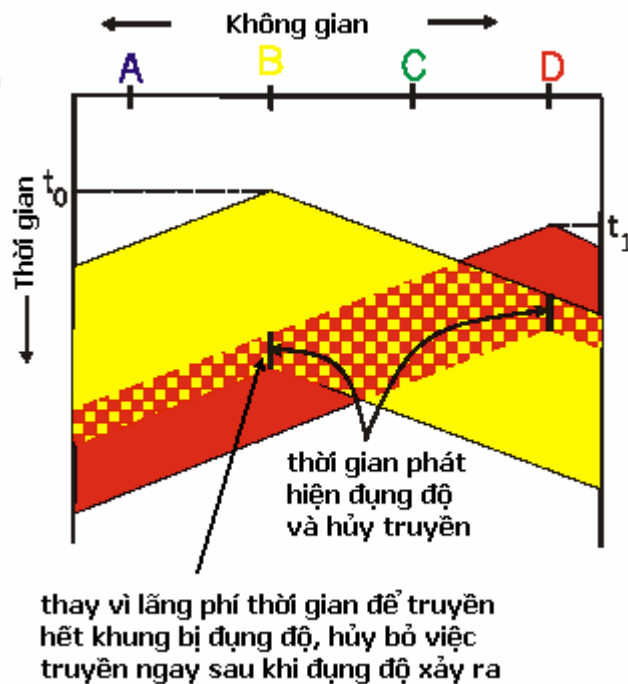
H5.13 Xử lý khu đụng độ
