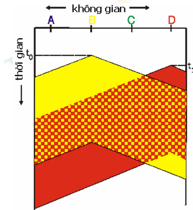
H5.9 Mô tả không gian và thời gian diễn ra đụng độ
