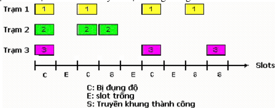
H5.7 Minh họa giao thức Slotted ALOHA
