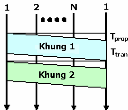
H5.19 Thời gian lan truyền và phát khung với RAR
