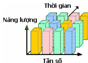
H5.6 Kết hợp giữa TDMA và FDMA
