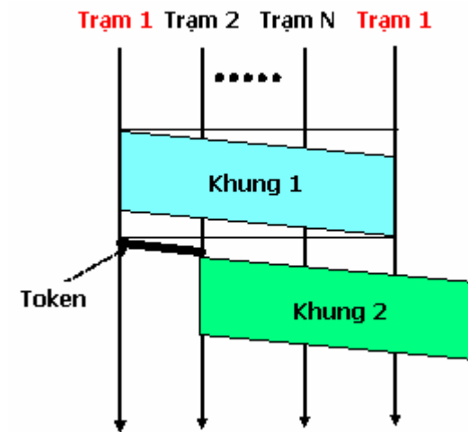
H5.18 Mô phỏng cơ chế chuyển thẻ bài trong RAR
