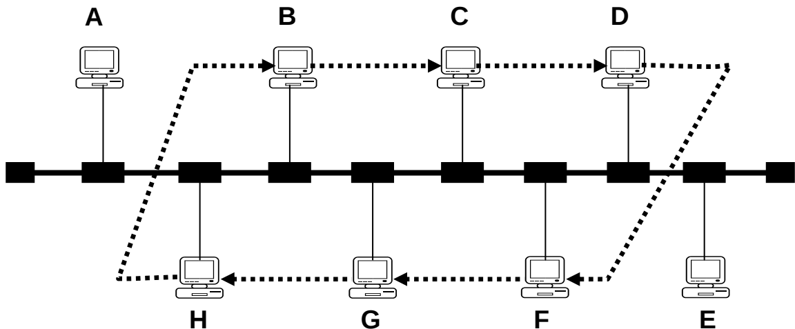
H5.24 Sơ đồ mạng Token Bus
