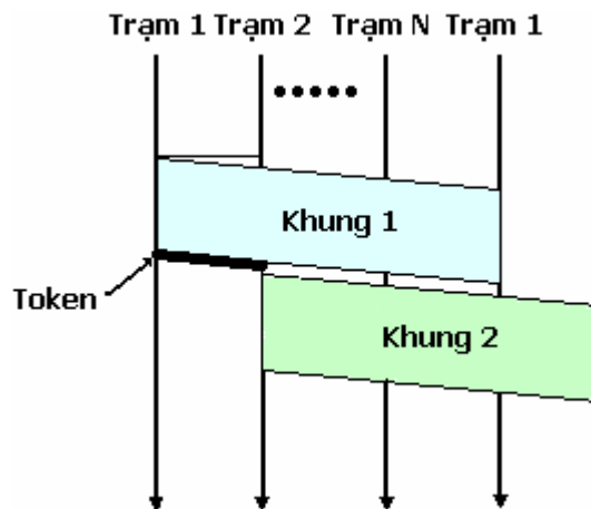
H5.21 Mô phỏng kỹ thuật RAT
