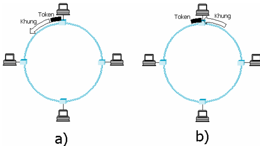
H5.16 Nhả token: a)RAT b)RAR
